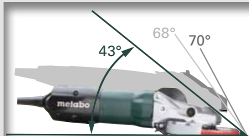
Mit patentierter Getriebebaumform: der Metabo Flachkopf-Winkelschleifer
